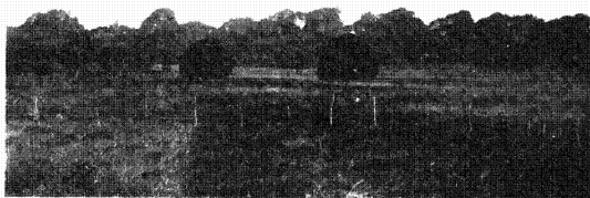
FIG. 3.— Haystack (pepino) hills
